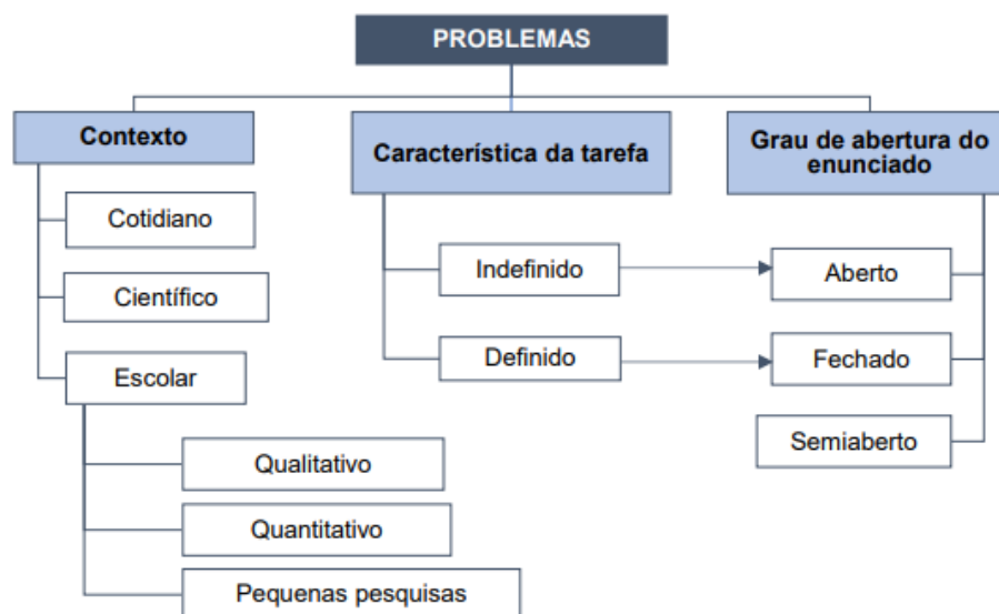
Figura 5: Tipologia dos Problemas.
