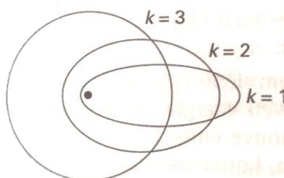
Figura 8: As órbitas de Bohr-Sommerfeld para n = 3 .
