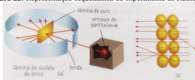
Figura 22: Representação esquemática do experimento de Rutherford.
